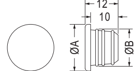
MOUNTING HOLE: ØG 【 MHD-17I 】
