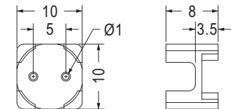
適用於 Ø10 的電容
