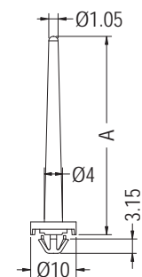
P.C.B Ø5.2 THICKNESS 0.6-0.8
