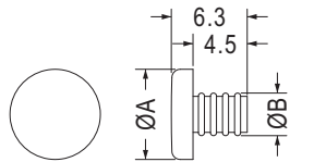
MOUNTING HOLE: ØG or M4 【 MHD-3.3 】
